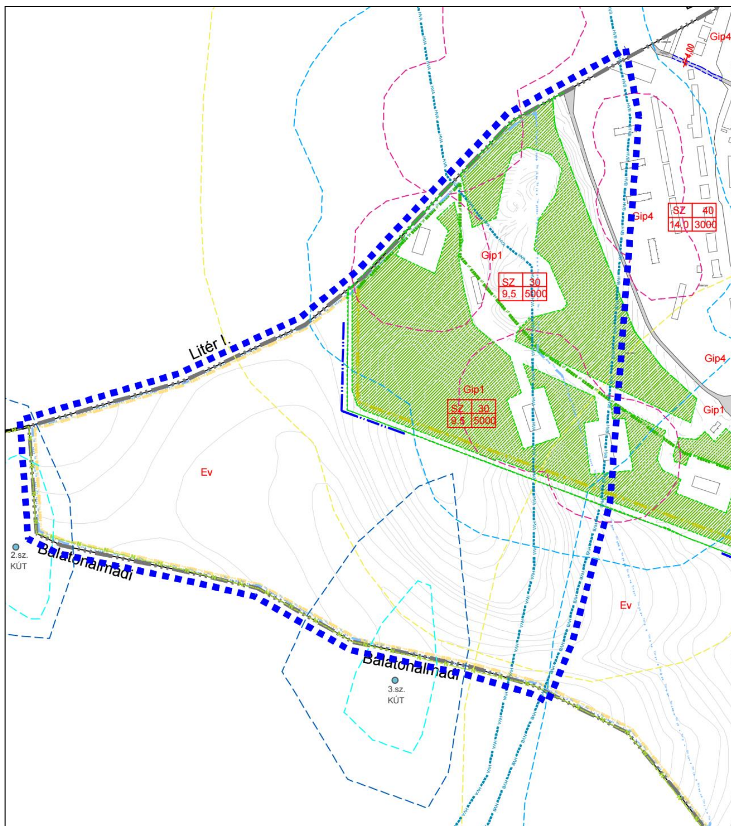
A Szabályozási terv 8m, 12 és 13 jelű szelvényének vonatkozó részlete (2. módosítás)
