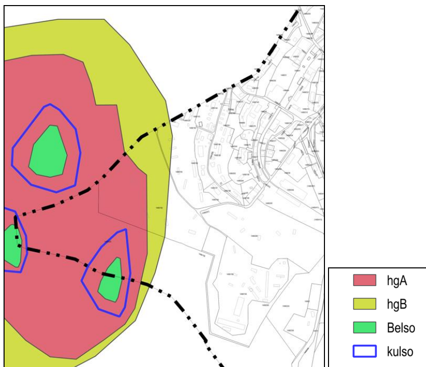
A kutak belső és külső védőidomai, és hidrogeológiai védőterületeinek elhelyezkedése
